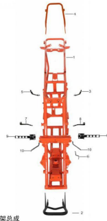
车架总成
