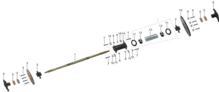
后桥总成
