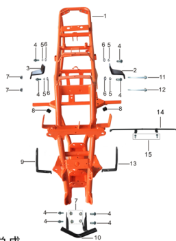
车架总成
