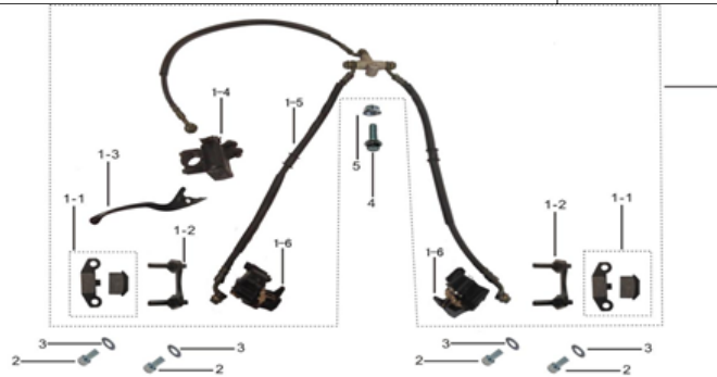
前制动总成
