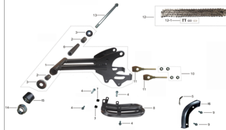
后平叉总成
