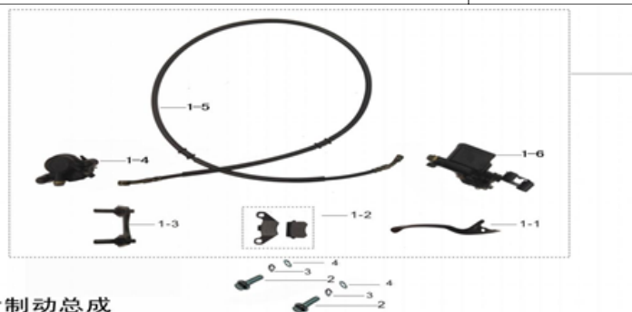
后制动总成
