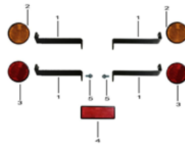
反射器
